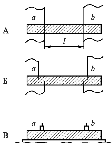
Рис. 1.9. Устройство для фиксации точек детонации: положение А – замкнутая цепь; положение Б – разомкнутая цепь; положение В – ионогазовая цепь
