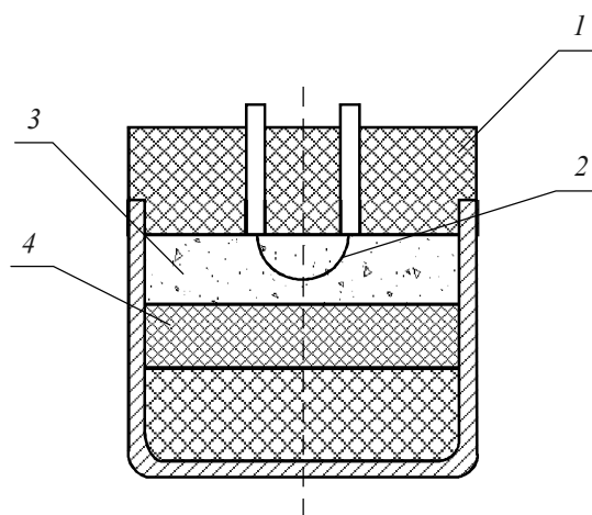
Рис. 5.4. Боеприпасные мостиковые электродетонаторы:
