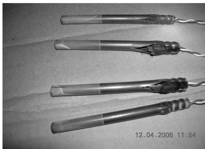
Рис. 9.10. Разрушение гильзы давлением продуктов горения замедляющего состава в зоне маркировки
