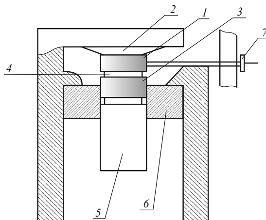
Рис. 1.16. Узел прибора Бодена–Козлова для определения чувствительности ВВ к трению:
