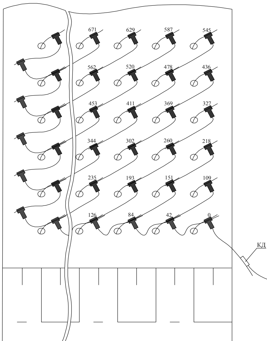
Рис. 9.12. Рабочие схемы взрывания скважинных зарядов неэлектрической системой «Искра» с поверхностным ( a ) и внутрискважинным ( б ) замедлением (см. также с. 294)
