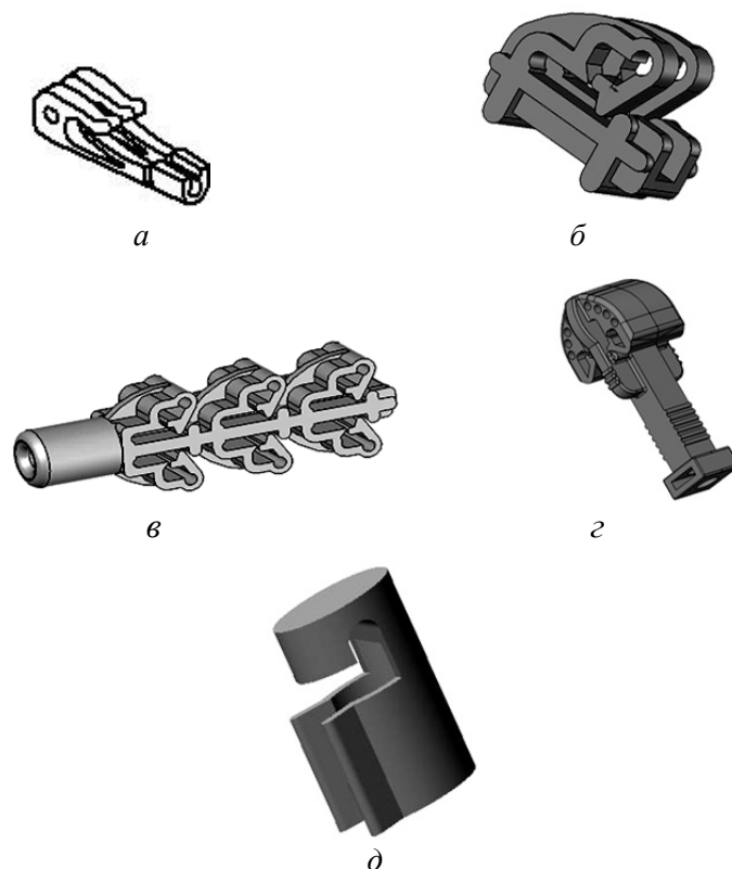
Рис. 9.4. Примеры соединителей системы «Искра»: a – соединитель (ДШ-1УВТ), ИВШП 143.000.000-02; б – соединитель (ДШ-3УВТ), ИВШП 313.000-01, -02; в – соединитель (монтажный блок ДШ-18УВТ), ИВШП 326.000; г – соединитель (ДШ-6УВТ), ИВШП 292.000; д – соединитель (ЗМВ-ДШ), ИВШП 331.000
