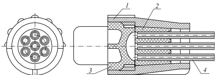
Рис. 9.25. Конструкция разветвителя:
