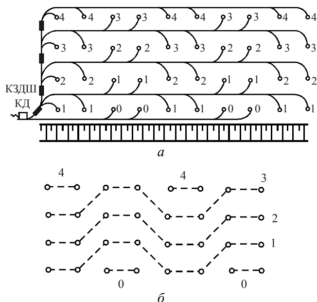
Рис. П5.3. Схема КЗВ с трапецевидными врубами: a – монтажная схема; б – последовательность действия взрыва зарядов
