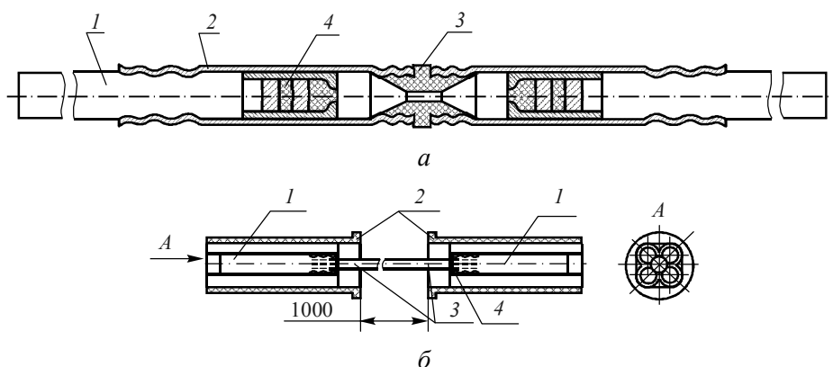
Рис. 9.2. Пиротехнические реле РП-Н (а) и РП-Д (б)
