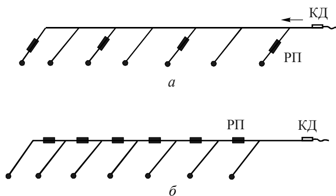
Рис. П5.1. Схемы однорядного КЗВ:
