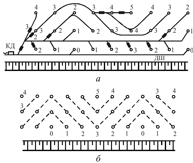
Рис. П5.4. Диагональная схема КЗВ с треугольными врубами:
