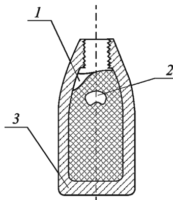
Рис. 7.1. «Перехват» и усадочная раковина при заливке:
