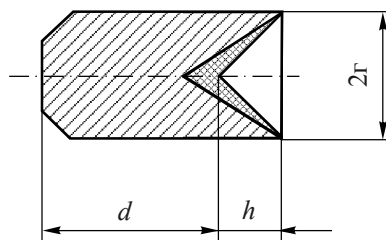
Рис. 2.8. НКЧ кумулятивного заряда
