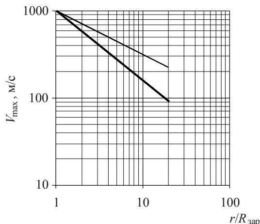
Рис. 9.22. Затухание волн напряжения в упругой среде и среде с трением: — упругая среда; — среда с трением
