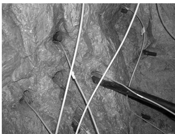
Рис. 9.7. Зарядание забоя пористой селитрой
