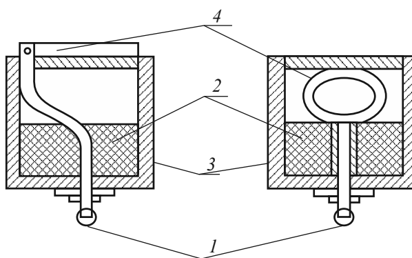
Рис. 4.2. Тёрочный капсюль-воспламенитель:
