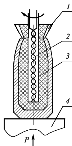
Рис. 7.7. Принцип шнекования:
