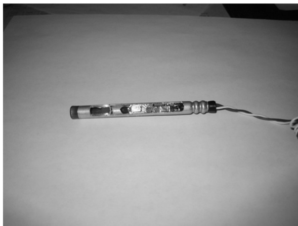
Рис. 9.6. Детонатор со встроенным сверхминиатюрным «интеллектуальным» микроконтроллером
