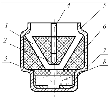
Рис. 4.8. Трубочный электрический капсюль-воспламенитель:
