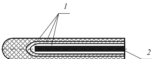
Рис. 5.6. Огнепроводный шнур:
