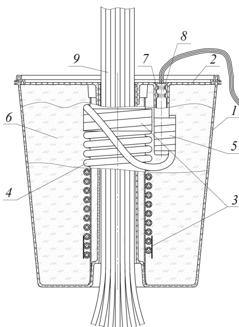
Рис. 9.16. Устройство УрсБ:
