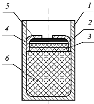
Рис. 5.2. Напольные капсулы-детонаторы:
