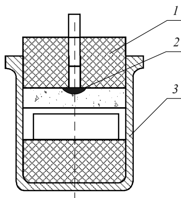
Рис. 5.5. Искровые электродетонаторы:
