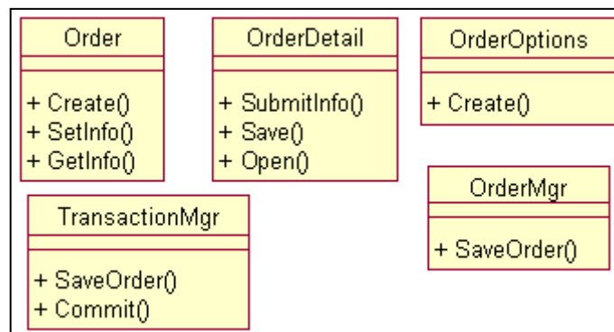
Рис. 2. Диаграмма классов для сценария "Ввести новый заказ"
